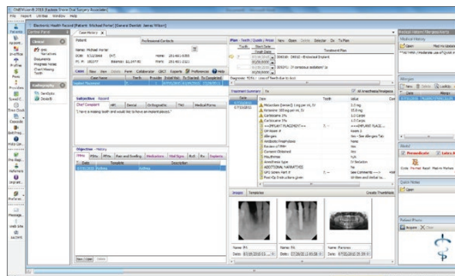
OMSVision EHR Main window.
